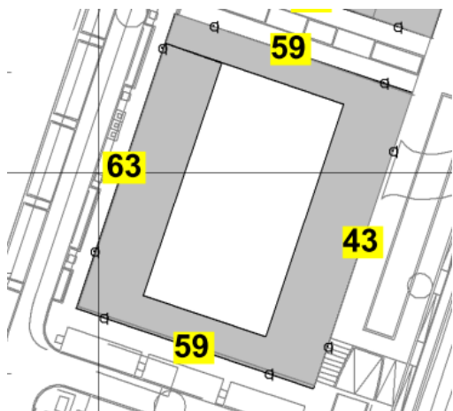
Figuur 5.3: Gecumuleerde geluidbelasting op basis van wegverkeerspectrum
